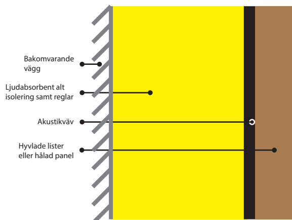
Genomskärning av ljudabsorberande vägg
